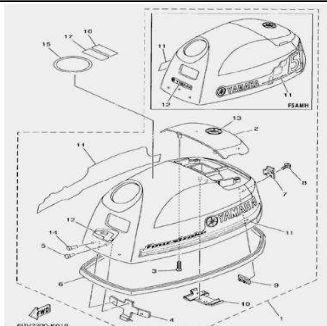
FIG. 1 TOP COWLING 顶罩总成
